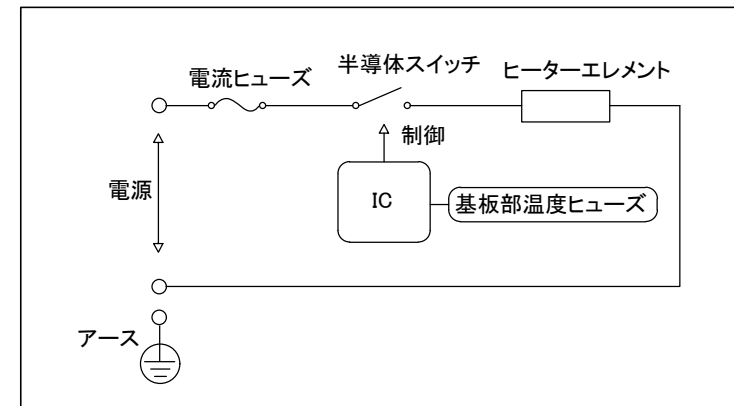
回路図(概略)
