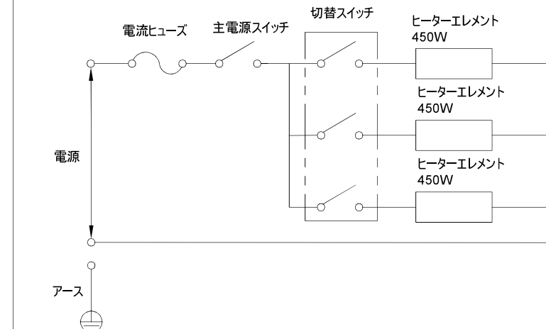
回路図(概略)
