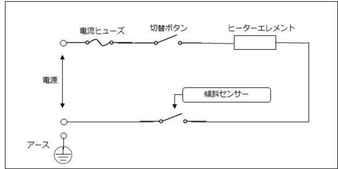
回路図 (概略)
