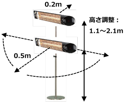
図：スタンド設置の場合の離隔距離
